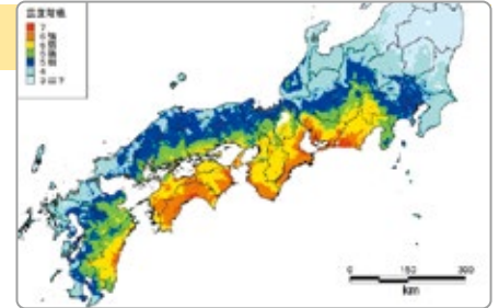
南海トラフ巨大地震の震度分布 (気象庁ホームページより)
